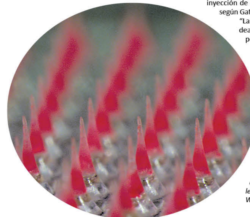
LA IMAGEN DEL MICROSCOPIO muestra microagujas de menos de un milímetro de altura que contienen el medicamento anticonceptivo levonorgestrel. (Foto: Wei Li, Georgia Tech)
